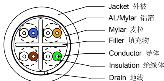
线材结构图
