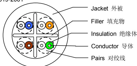
线材结构图(加十字架)
