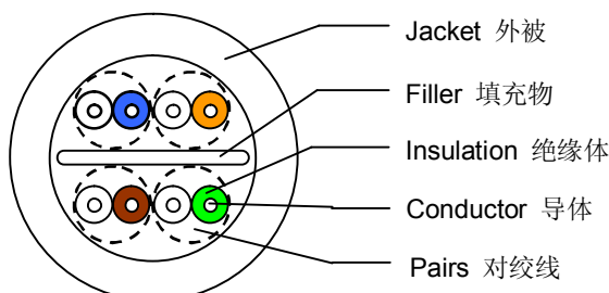
线材结构图(加发泡薄片)
