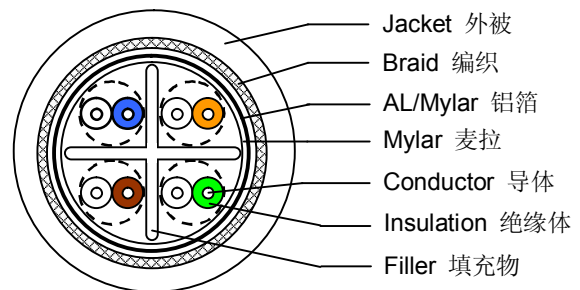
线材结构图
