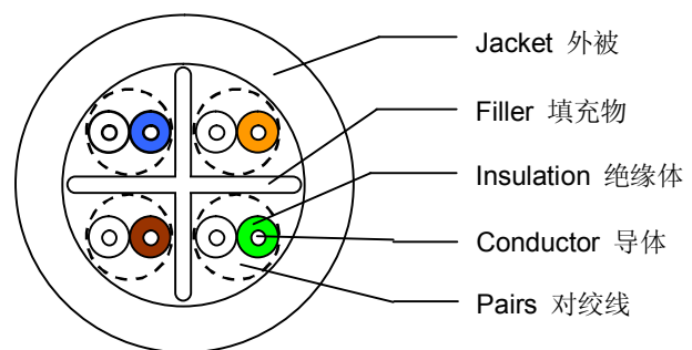
线材结构图
