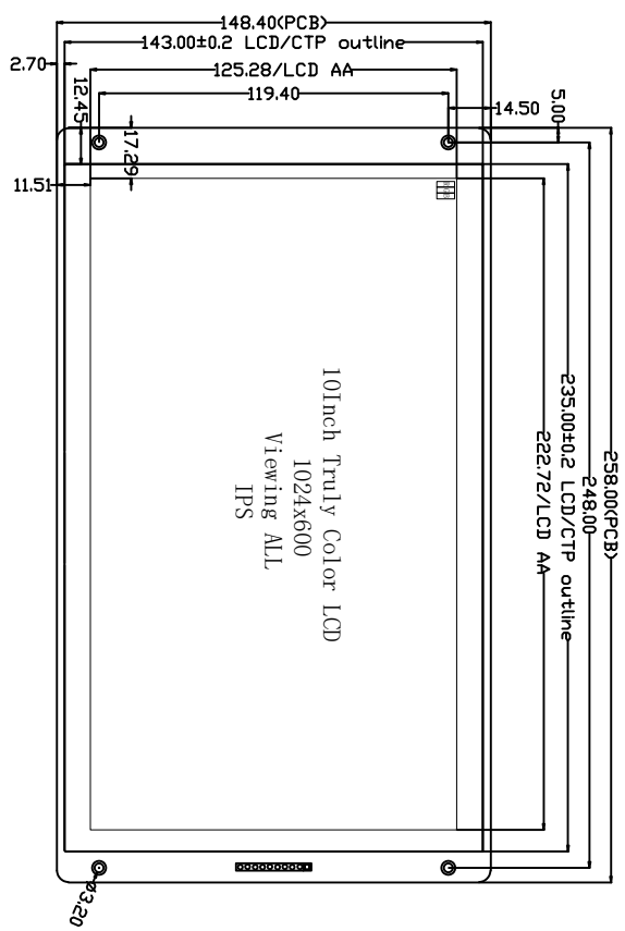
正视图
