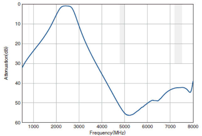
□ ATTENUATION
