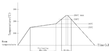
SMT 回流焊
