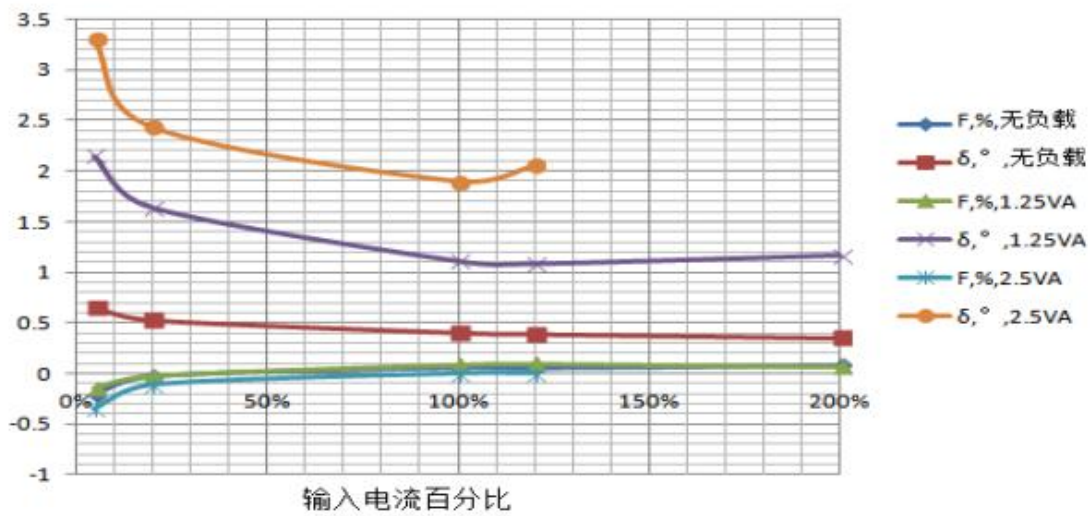
[ 400A/1A 不同负载性能曲线 ]
