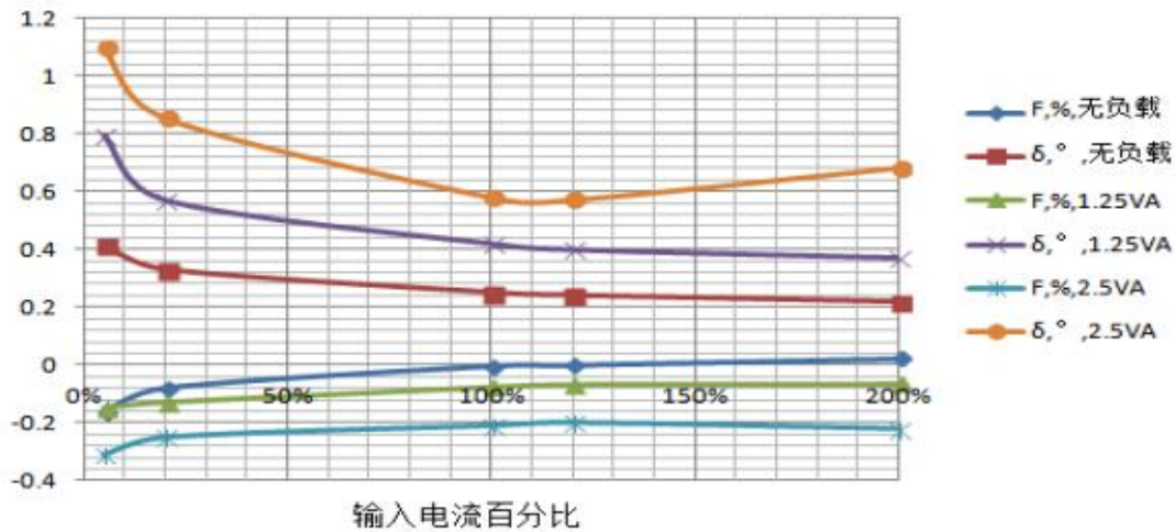
[ 400A/1A 不同负载性能曲线 ]
