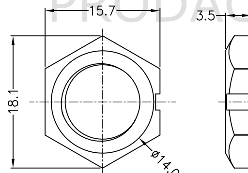
HEX NUT
