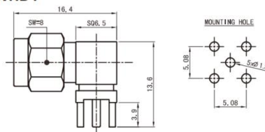
SMA-50JWHD4
