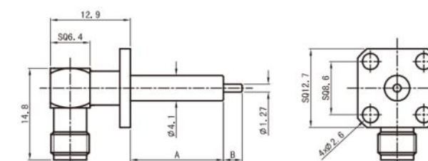
SMA-50KWFD
