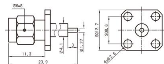
SMA-50JWHD4
