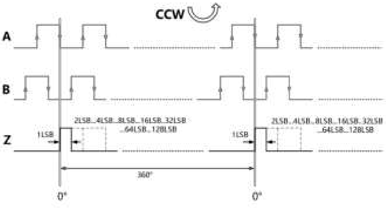
Figure 11: Typical ABZ Output with Z pules width =1、 2、 4、 8、 16、 32、 64、 128LSBs
